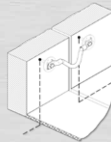
Anwendungsbild 2: Überbrückung von Bewegungsfugen außerhalb des Betons
