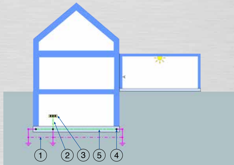
Bild 14: Teilunterkellertes Gebäude ohne Erdungsanlage im Nebengebäude
