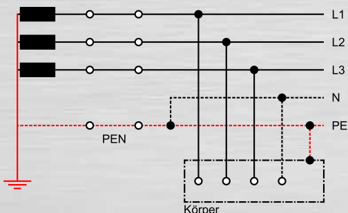
TN-C-S-System
