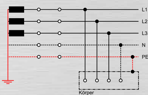
TN-S-System
