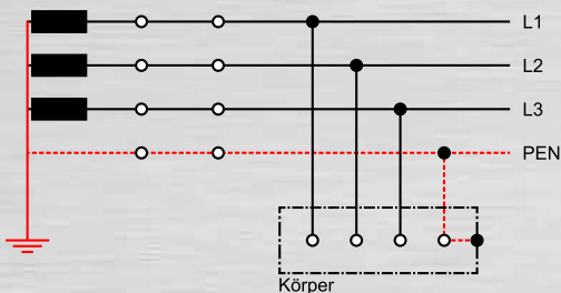
TN-C-System
